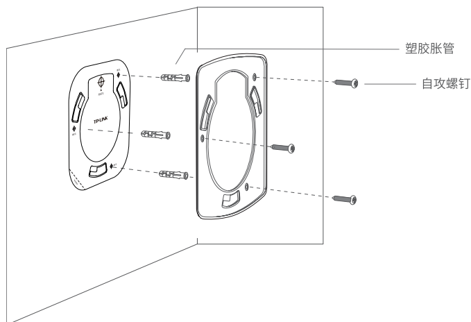
图3-10 固定安装架到墙面示意图
