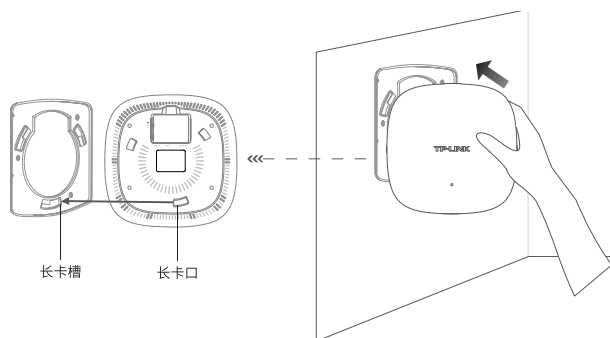
图3-11 安装AP到安装架示意图
