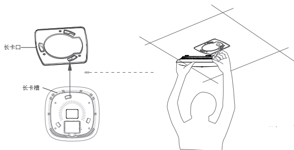
图3-5 安装AP到安装架示意图
